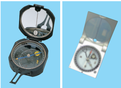
ブラントンコンパス
